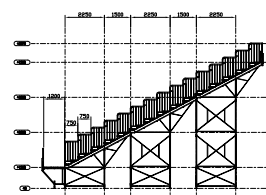
SEZIONE LATERALE TIPICA LATO PARAPETTI
