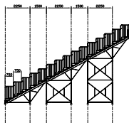
SEZIONE LATERALE TIPICA LATO PARAPETTI
