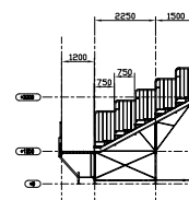
SEZIONE LATERALE TIPICA LATO PARAPETTI
