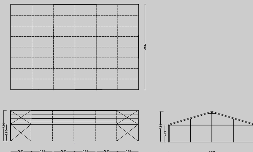
TENDOSTRUTTURA DOPPIA FALDA ARCATA 20 MT ALTEZZA IN GRONDA MT 3/4
