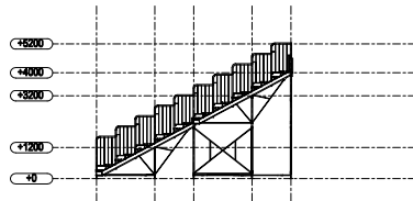
SEZIONE LATERALE TIPICA LATO PARAPETTI
